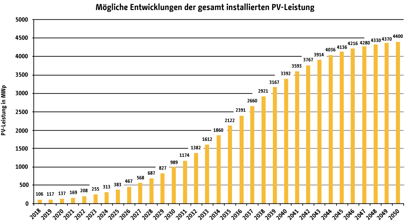
Abb. 3: Im Masterplan Solarcity skizzierte mögliche Entwicklungen der gesamten installierten PV-Leistung
